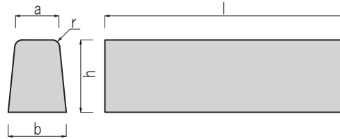
■両面歩車道境界ブロック (JIS A 5371)
