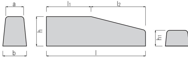
■歩車道境界ブロック 歩道乗り入れ部
