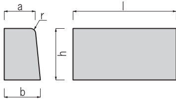
■地先境界ブロック (JIS A 5371)
