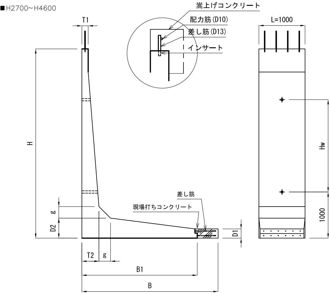
嵩上擁壁（CL嵩上擁壁嵩上400）規格表
