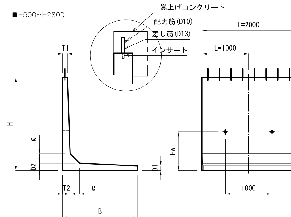
嵩上擁壁（CL嵩上擁壁）規格表
