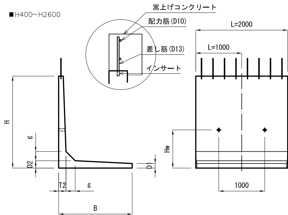
嵩上擁壁（CL嵩上擁壁嵩上400）規格表
