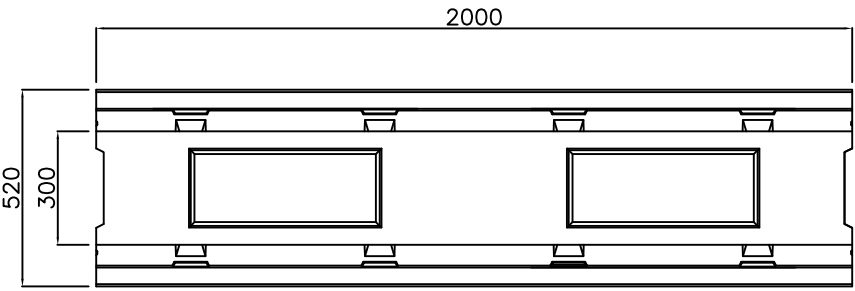
平面図
