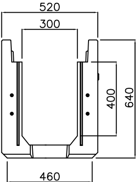
正面図
