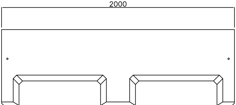
側面図
