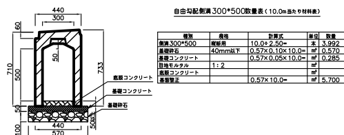
自由勾配側溝 300*500 (縦断用)
