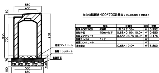
自由勾配側溝 400*700 (縦断用)
