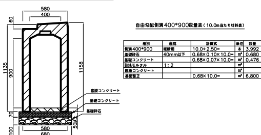
自由勾配側溝400*900(縦断用)
