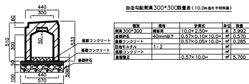
自由勾配側溝300*300(縦断用)
