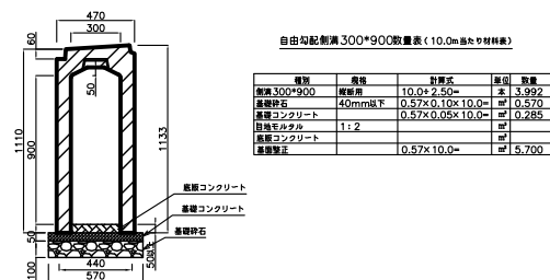
自由勾配側溝300*900(縦断用)
