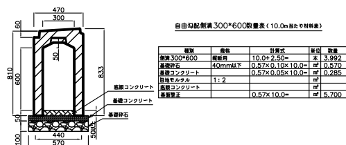
自由勾配側溝300*600(縦断用)
