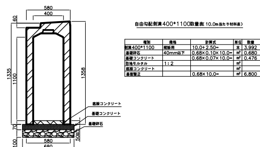
自由勾配側溝 400*1100 (縦断用)
