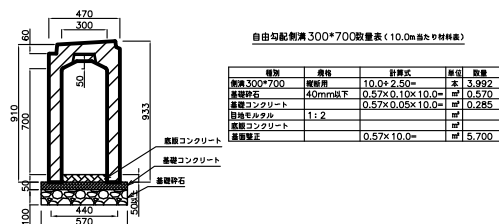
自由勾配側溝300*700(縦断用)
