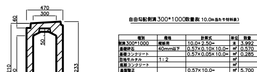
自由勾配側溝 300*1000 (縦断用)
