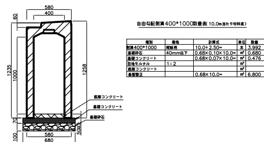
自由勾配側溝 400*1000 (縦断用)
