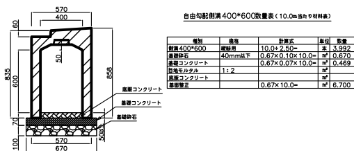
自由勾配側溝 400*600 (縦断用)
