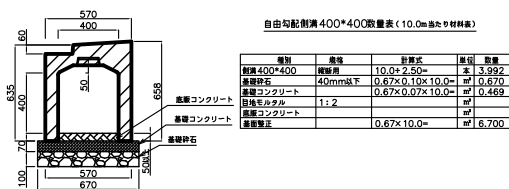
自由勾配側溝 400*400 (縦断用)
