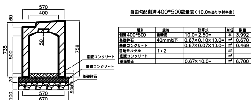
自由勾配側溝400*500(縦断用)
