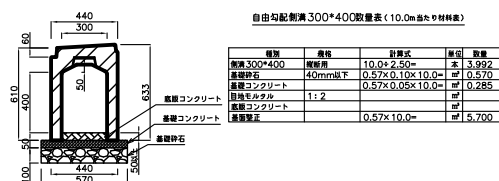
自由勾配側溝300*400(縦断用)
