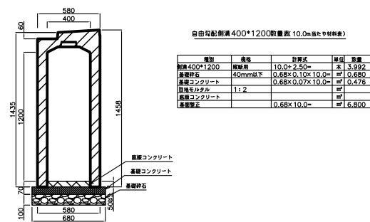
自由勾配側溝 400*1200 (縦断用)
