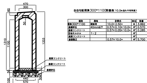
自由勾配側溝300*1100(縦断用)
