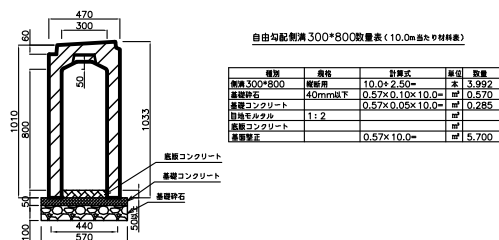
自由勾配側溝300*800(縦断用)
