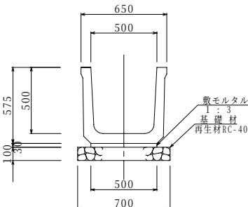
標準断面図 KD-500
