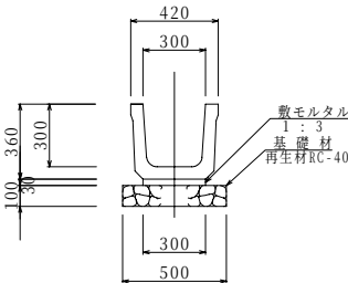
標準断面図 KD-300
