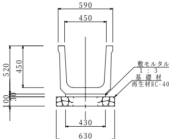
標準断面図 KD-450
