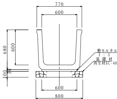
標準断面図 KD-600
