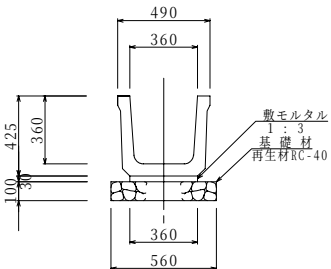
標準断面図 KD-360
