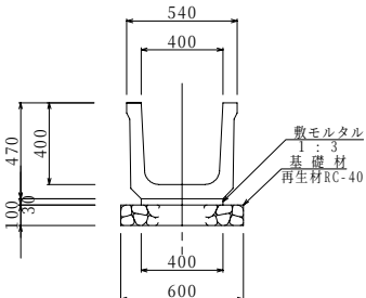
標準断面図 KD-400
