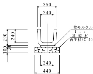
標準断面図 KD-240
