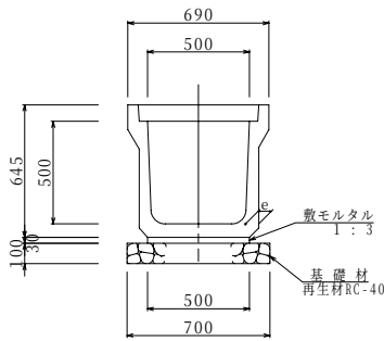
標準断面図 AT500型
