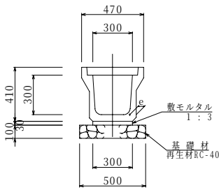
標準断面図 AT300型
