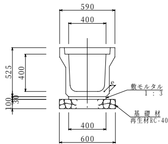
標準断面図 AT400型
