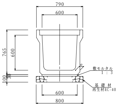
標準断面図 AT600型
