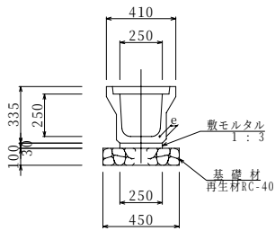
標準断面図 AT250型
