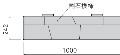
■平面図
