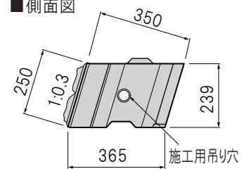
■側面図
